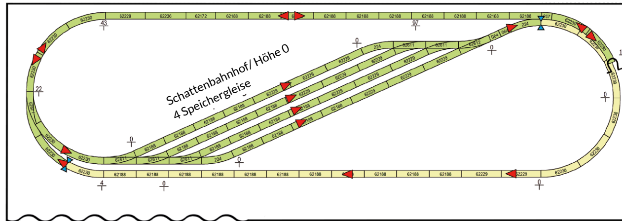
Zweiter Schattenbahnhof, Höhe 0, 4 Speichergleise
