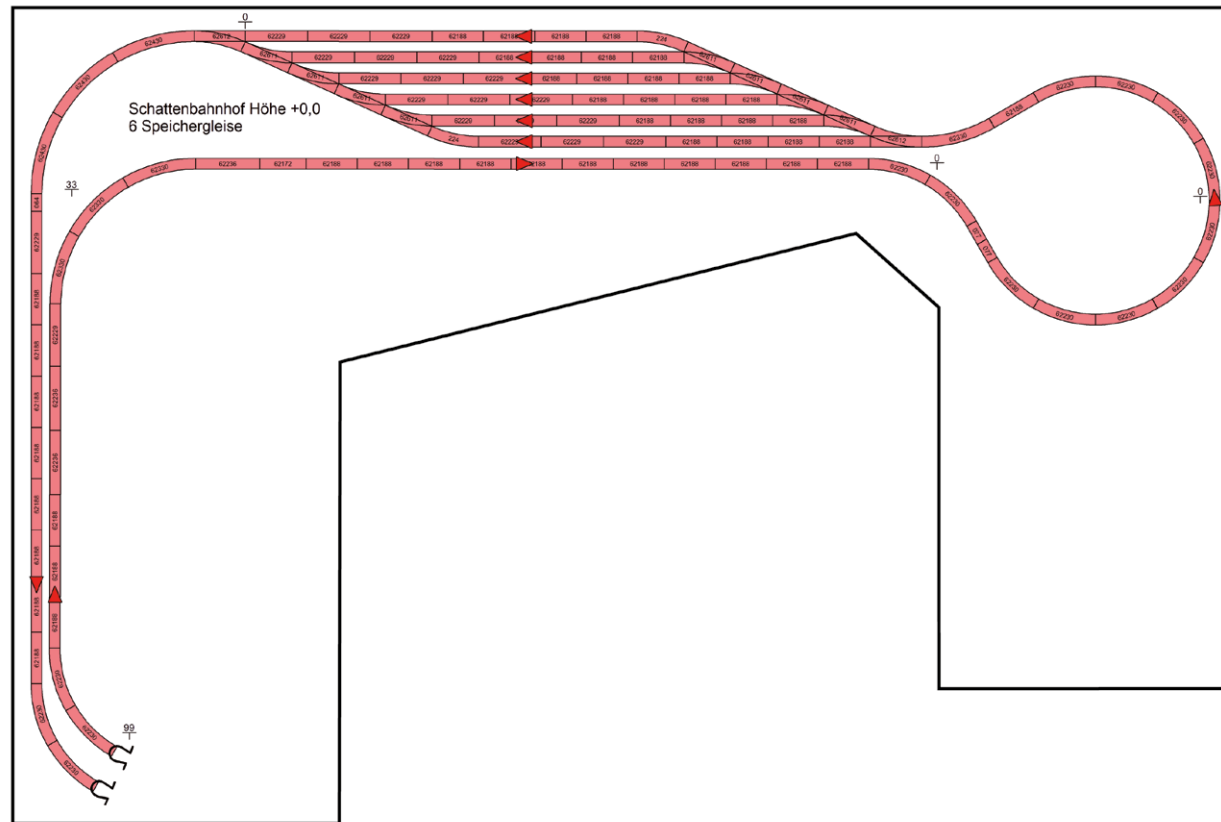
Erster Schattenbahnhof, Höhe 0
