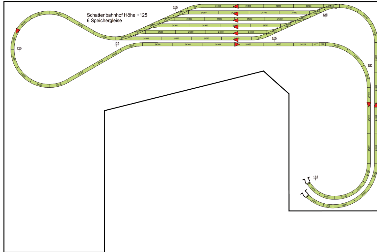
Zweiter Schattenbahnhof, Höhe +125
